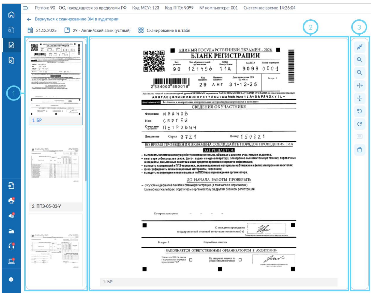
Рис. 7.19. Режим подробного просмотра изображений
