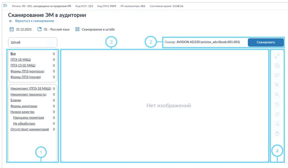
Рис. 7.11. Страница «Сканирование ЭМ в аудитории», сканирование не начиналось Страница «Сканирование ЭМ в аудитории» состоит из следующих блоков:
