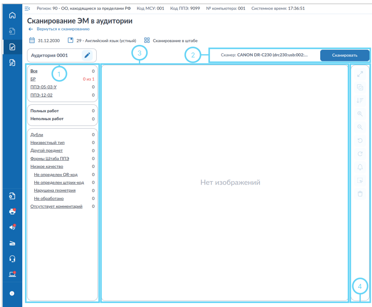
Рис. 7.15. Страница «Сканирование ЭМ в аудитории», устный экзамен по иностранному языку, сведения об аудитории введены, сканирование не начиналось
