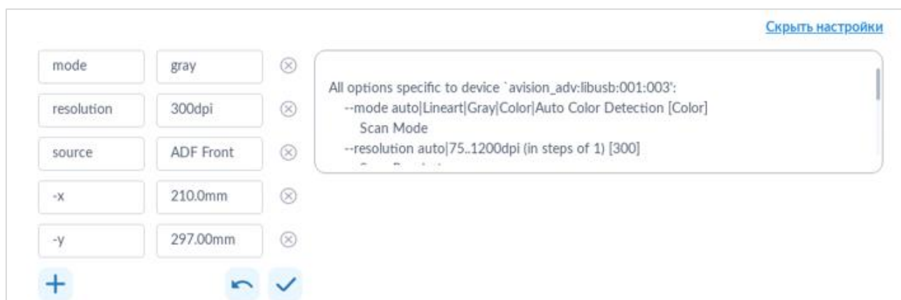
Рис. 3.18. Пример указания параметров сканирования
